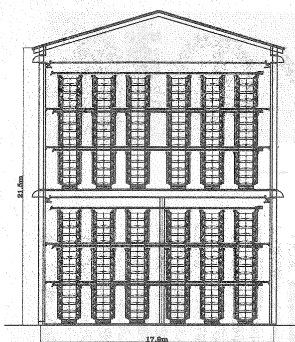
12段6列2階建て鶏舎の断面図。換気は夏冬切り替え3分割インレットを特長とするハイテム新トンネル換気
